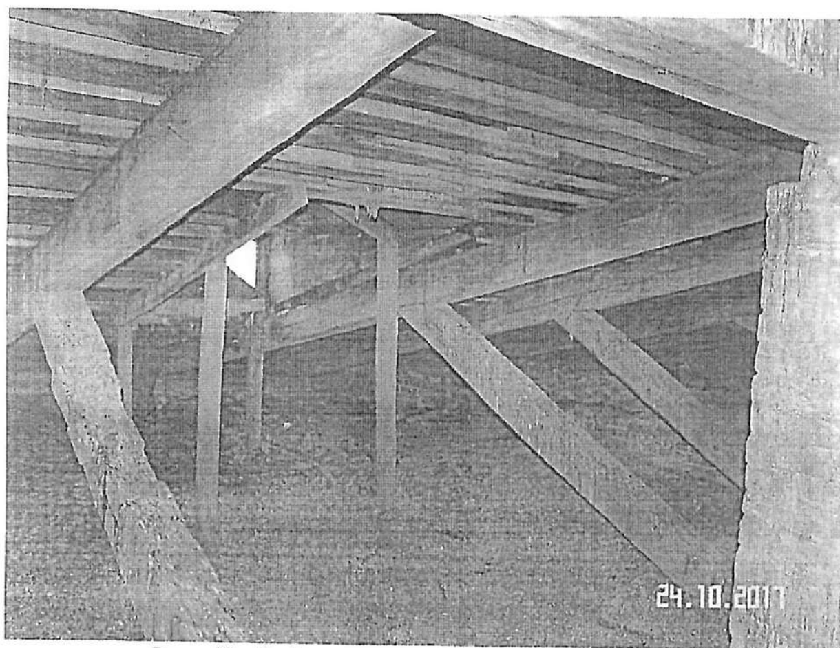
Фото 47, 48. Состояние стропильных конструкций.
