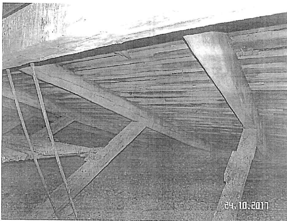
Фото 45, 46. Состояние стропильных конструкций.
